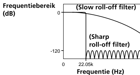
Vergelijking tussen de scheidingskarakteristieken van een sharp roll-off filter en slow roll-off filter
